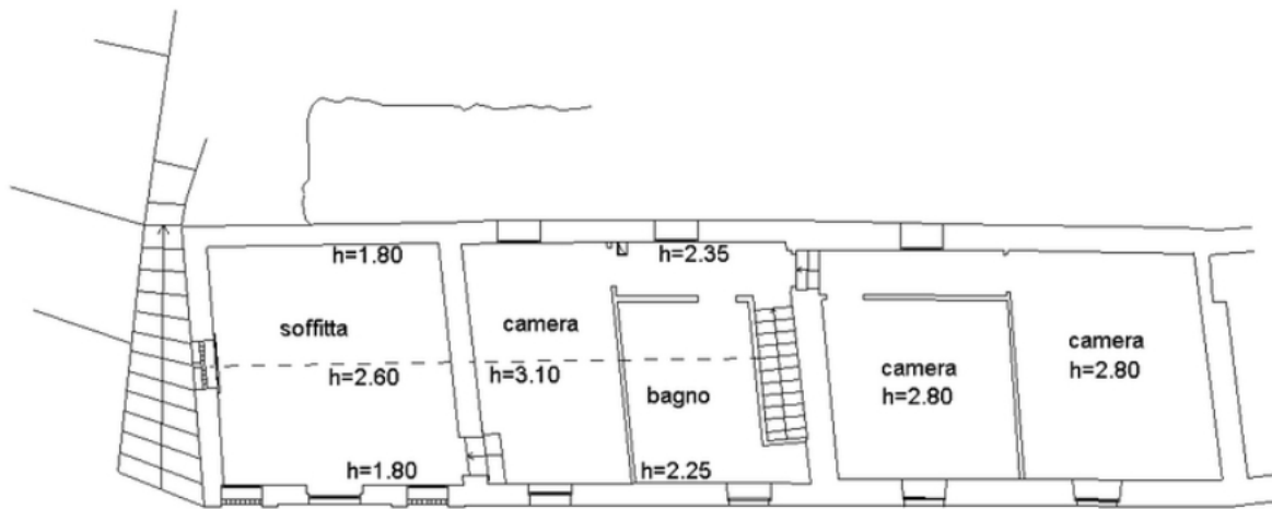
PIANO PRIMO
